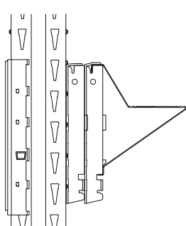
20 Guida DRIVE-IN su staffa singola e doppia
