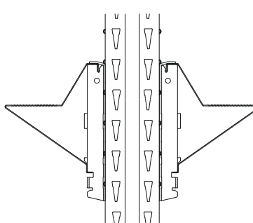
21 Guida DRIVE-IN bifronte su staffa singola
