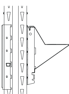
20 Guida DRIVE-IN su staffa singola e doppia
